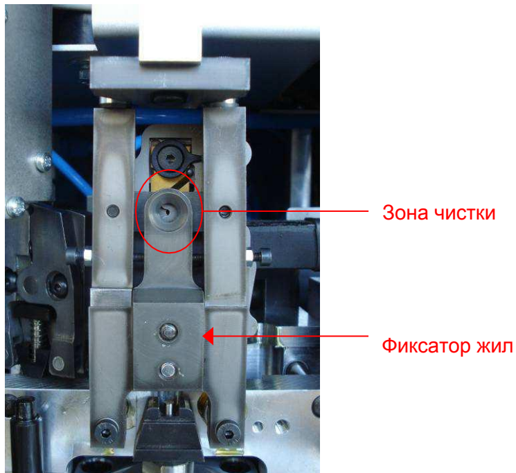
Рис. 6: Фиксатор жил
