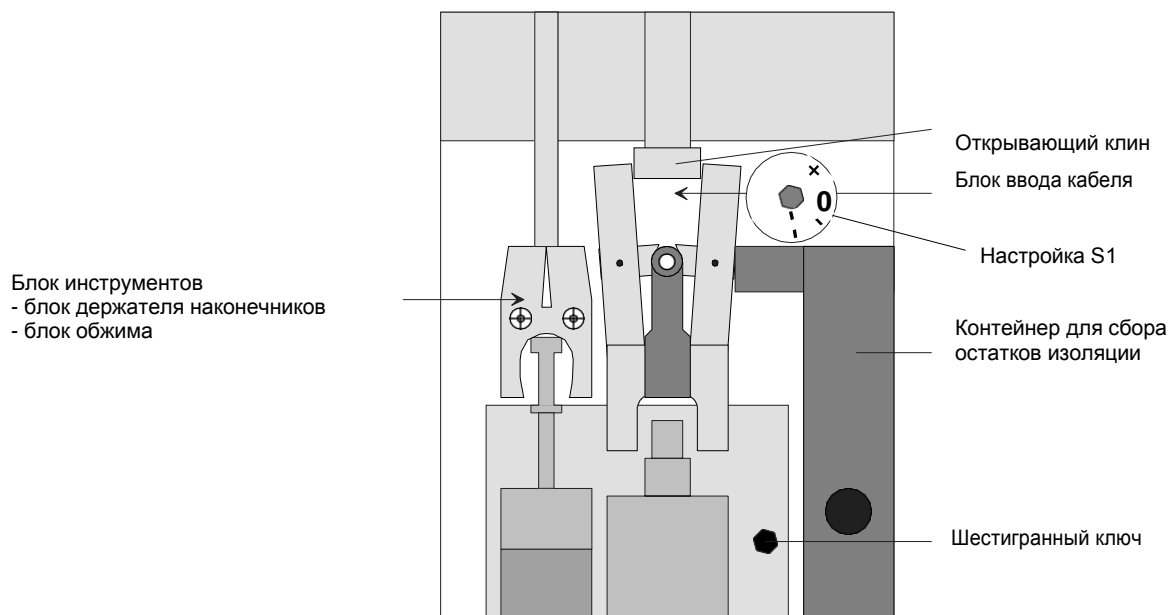
Рис. 1: Вид изнутри
